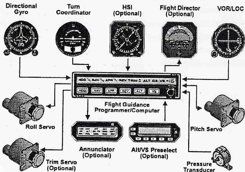
Schéma du Pilote Automatique S-TEC System 55.
